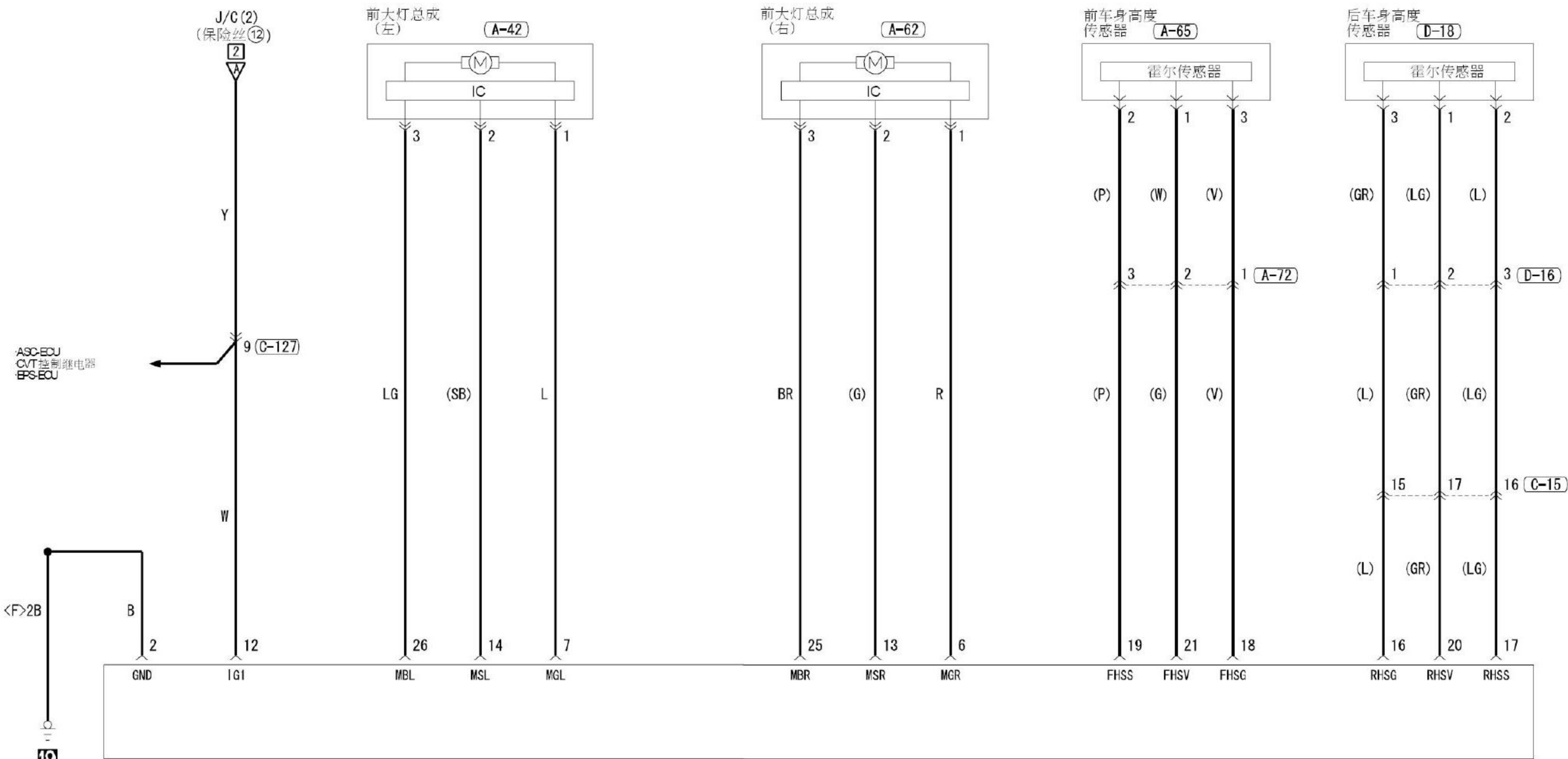
前大灯自动调平-ECU (C-117)
